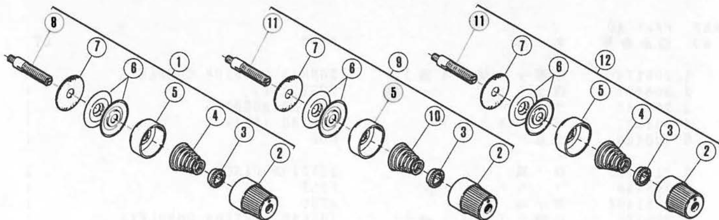
L52・1本針 1-needle L52
