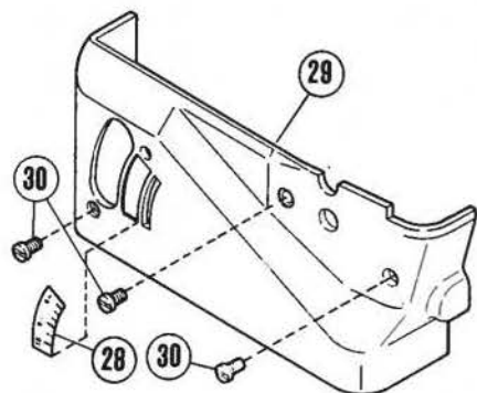
L52 クロスプレート狭巾用 For cloth plate (narrow)
