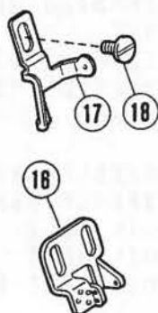
L52・2本針 2-needle L52
