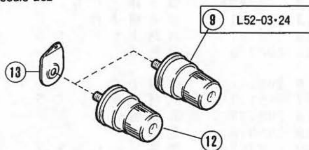
L52・2本針 2-needle L52
